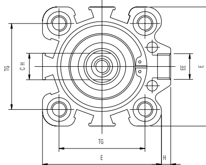
Ø 32-40-50-63-80-100
